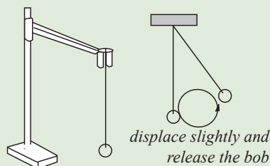
Fig. 7.4: Simple pendulum
