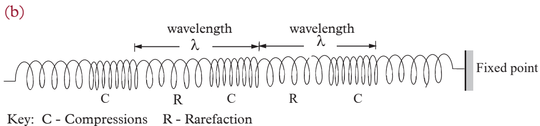
Fig. 7.12: Longitudinal wave
