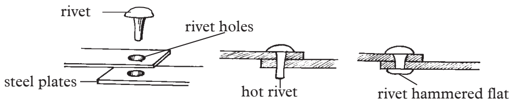
Fig. 9.27: Rivets
